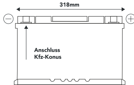
Abmaße: Länge 318mm | Breite 175mm | Höhe 190mm
