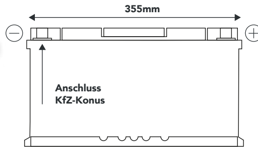
Abmaße: Länge 355mm | Breite 175mm | Höhe 190mm
